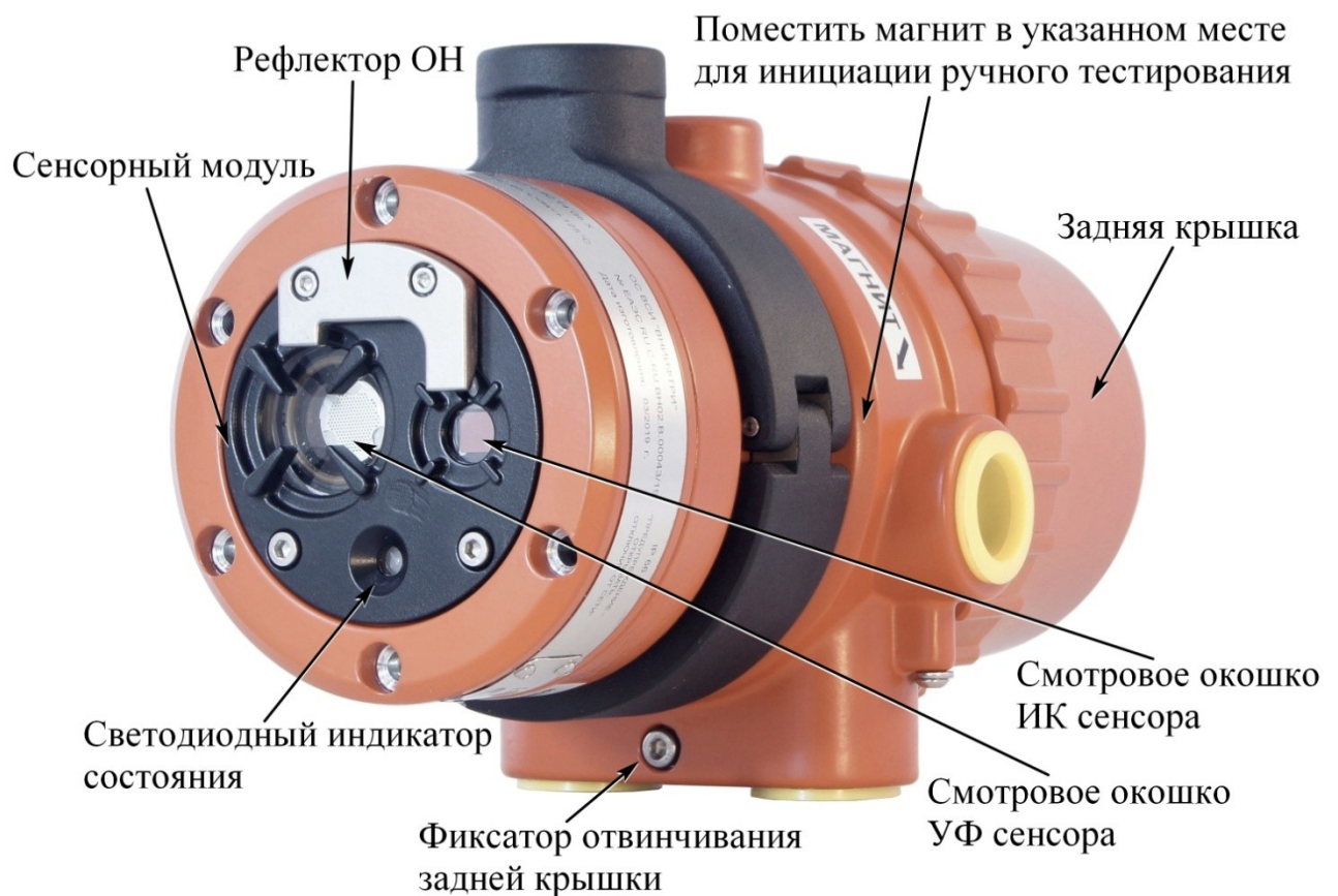
Рисунок 1 – Общий вид извещателя «СПАРК» ИП 329/330-20
