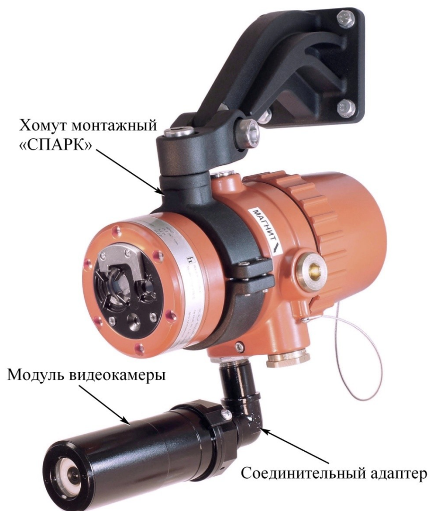
Рисунок 3 – Извещатель «СПАРК» ИП 329-20 с видеокамерой.
