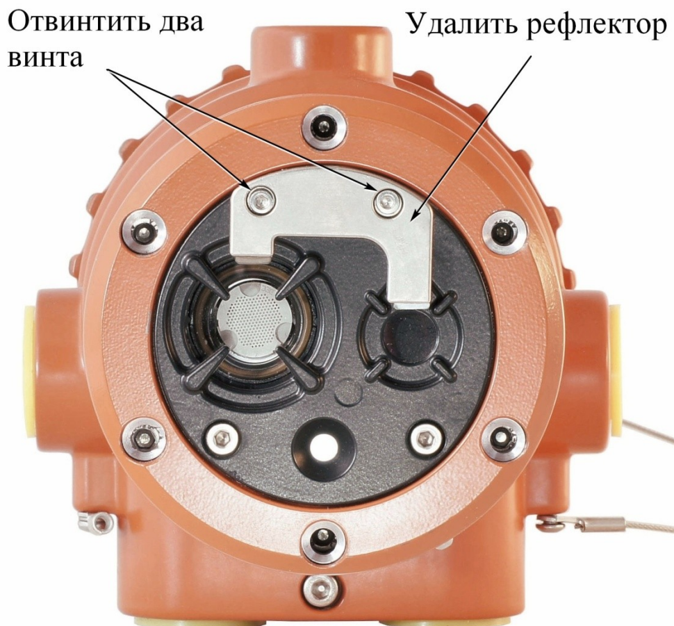
Рисунок 19 — Снятие рефлектора ОН.
