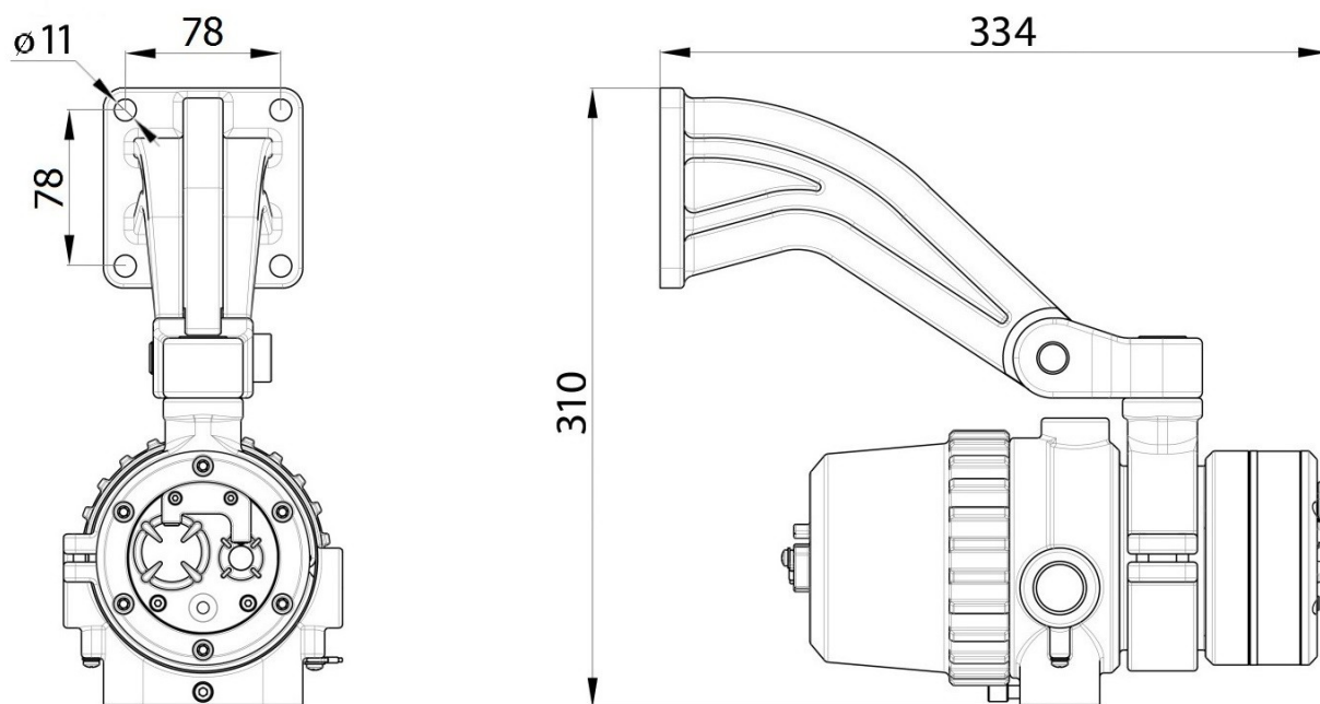
Рисунок 7 – Габаритные размеры извещателя «СПАРК» ИП 329-20 с кронштейном монтажным извещателей пламени «СПАРК» и хомутом монтажным «СПАРК»
