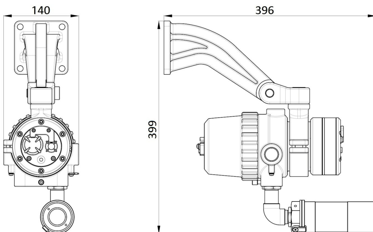
Рисунок 7а– Габаритные размеры извещателя «СПАРК» ИП 329-20 с видеокамерой, кронштейном монтажным извещателей пламени «СПАРК» и хомутом монтажным «СПАРК»
