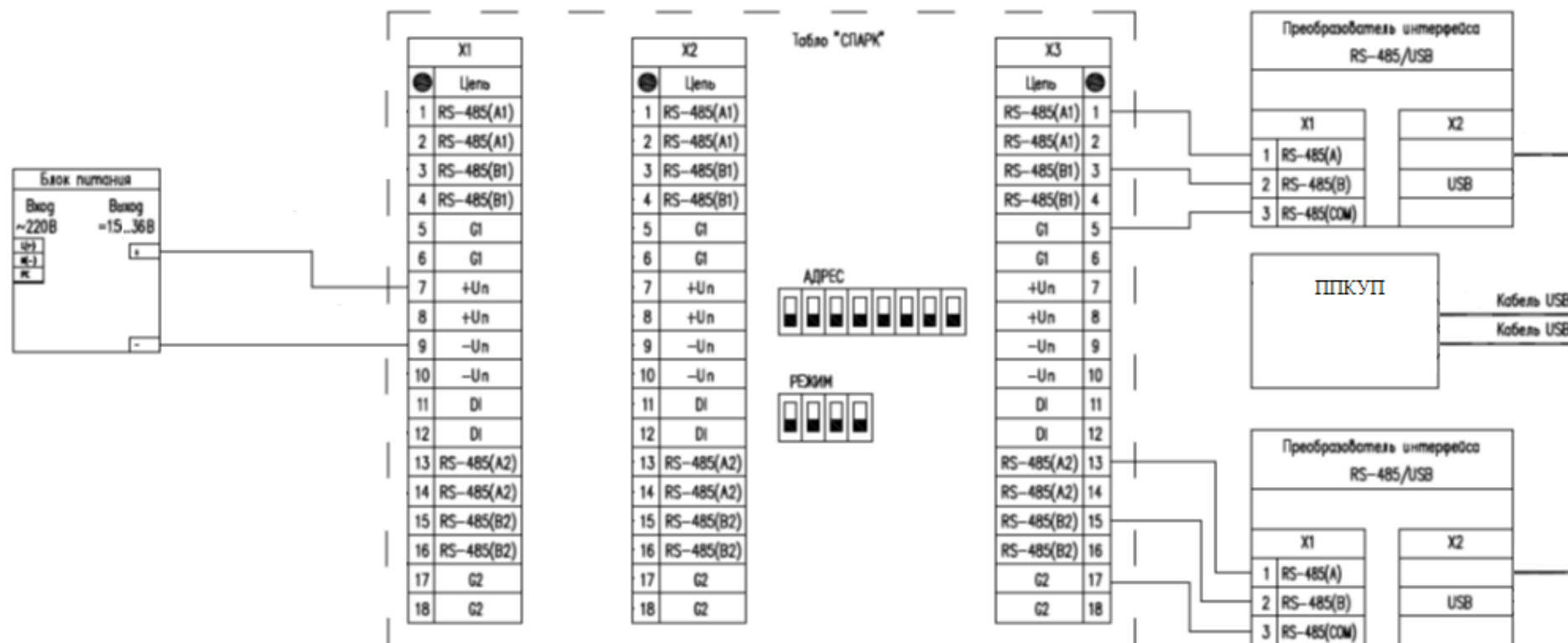
Рисунок Б.1 - Схема подключения табло.
