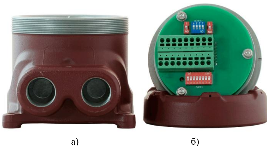
Рисунок 2 - Внешний вид извещателя со стороны резьбовых отверстий и клеммных разъемов
