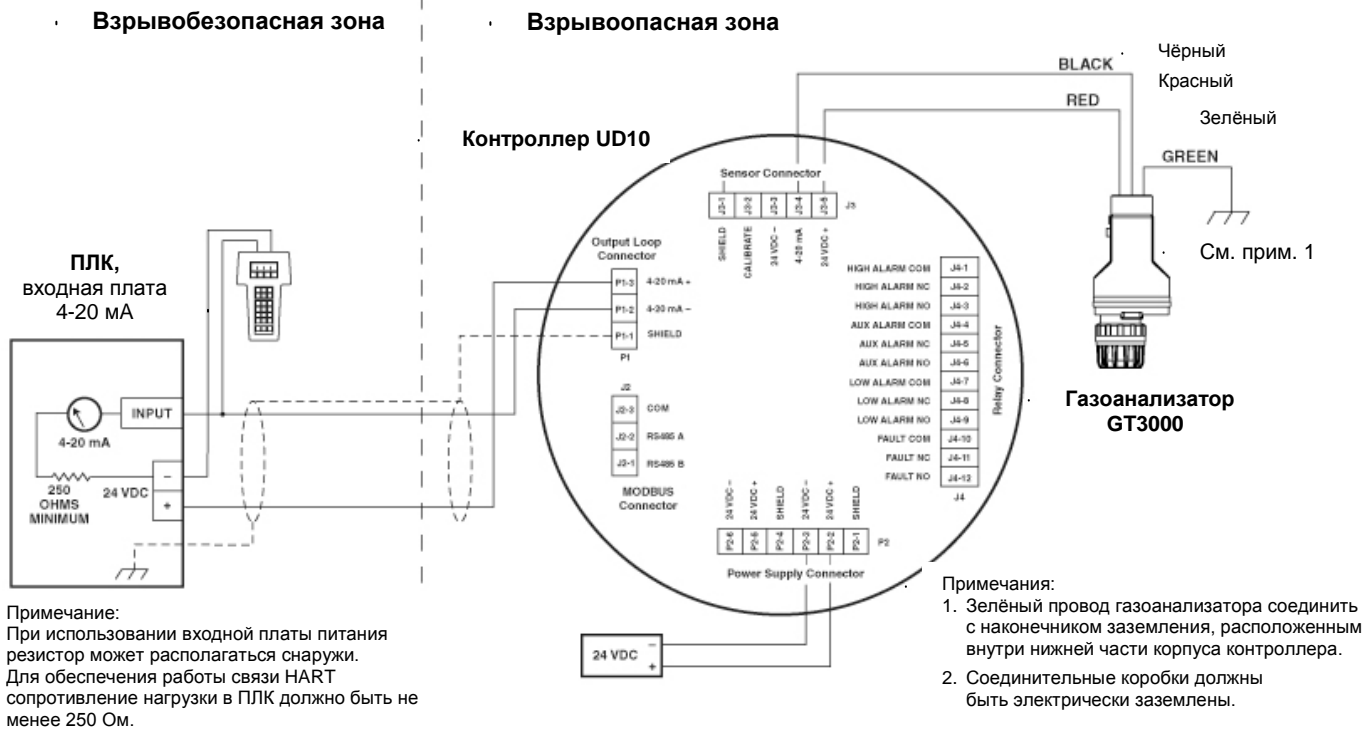
Рис. 12. Газоанализатор GT3000, подключенный непосредственно к контроллеру UD10, и контроллер UD10, соединённый с ПЛК через изолированный выход 4-20 мА.
