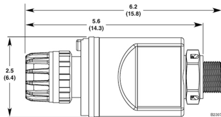
Рис. 1. Габаритные размеры газоанализатора GT3000 в дюймах (см).
