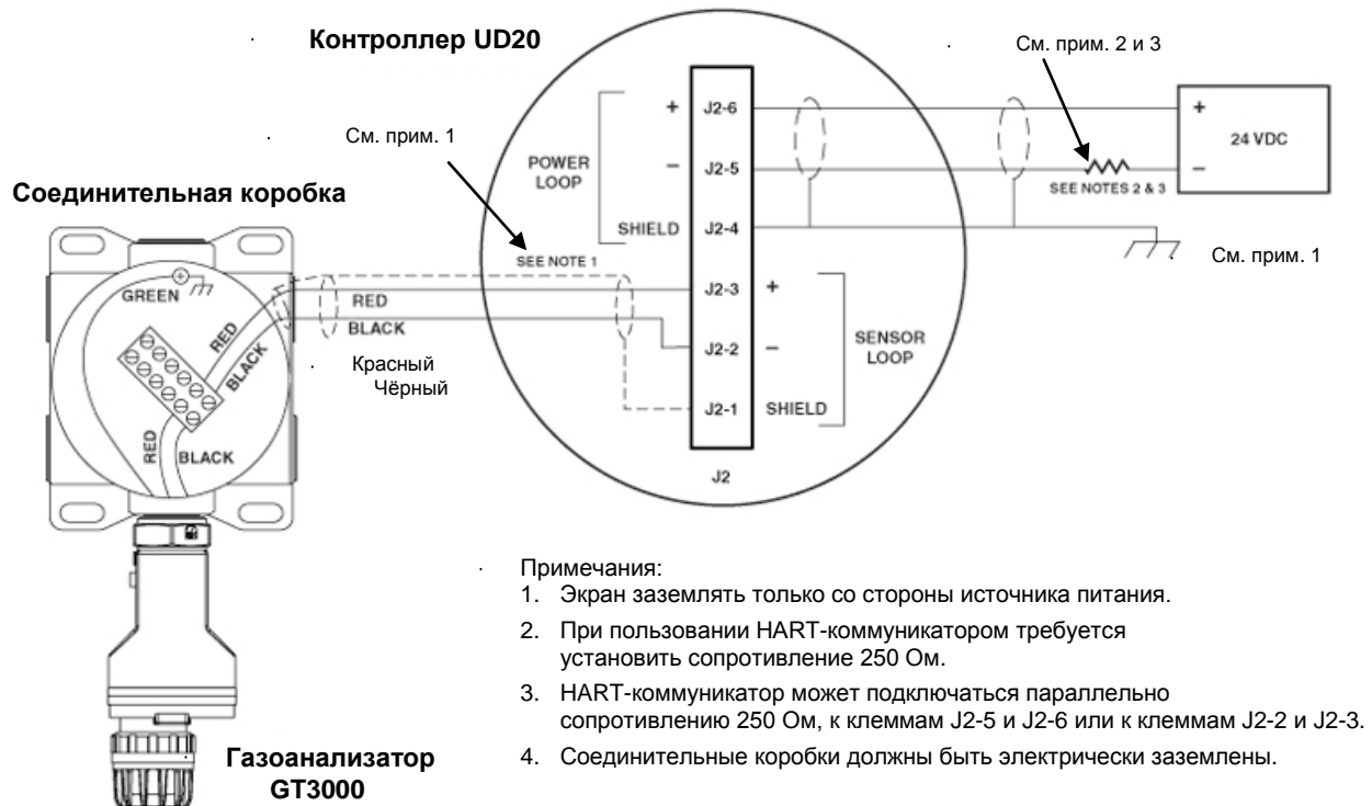
Рис. 9. Газоанализатор GT3000, подключенный к контроллеру UD20 через соединительную коробку.
