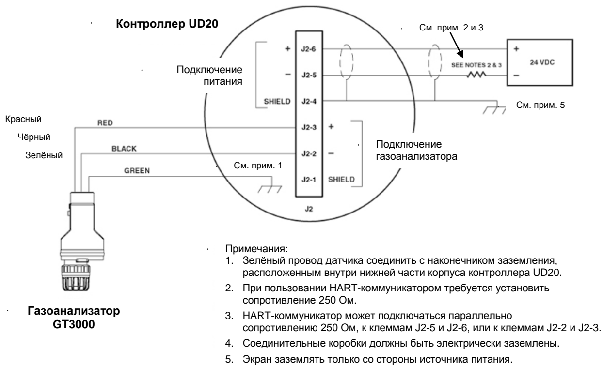
Рис. 8. Газоанализатор GT3000, подключенный непосредственно к контроллеру UD20.
